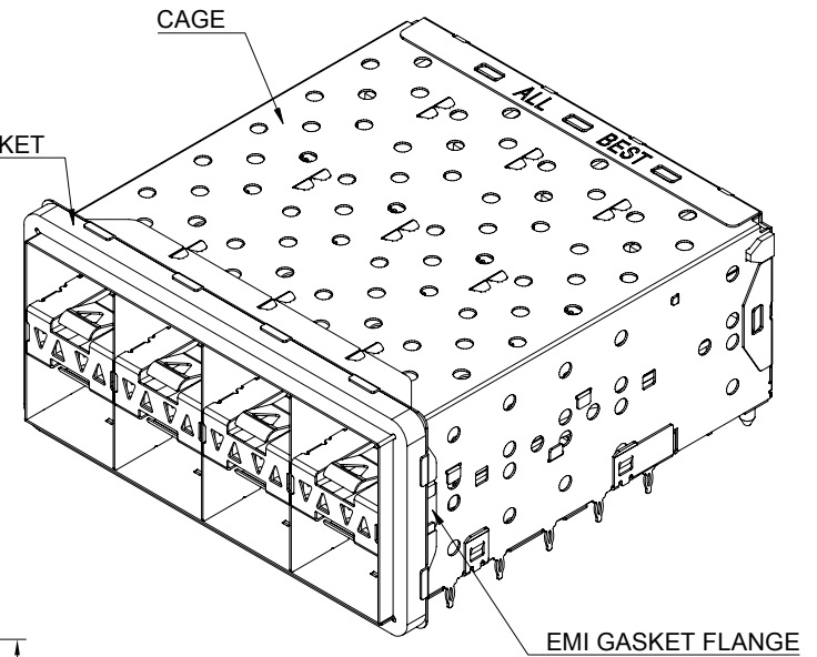
EMI GASKET FLANGE
